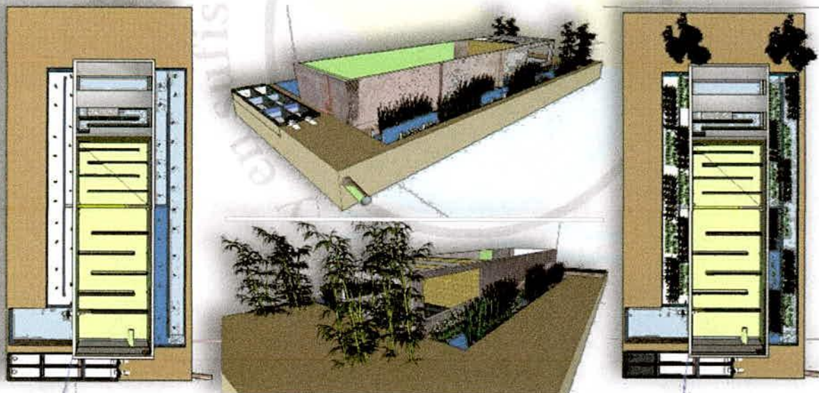
Imagen 4. Diseño de adecuación a la fosa séptica de la localidad de La Laja, municipio de El Grullo, para convertirla en humedal de tratamiento de aguas residuales.
